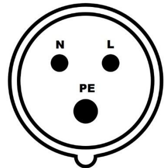
Steckdose Typ 23
